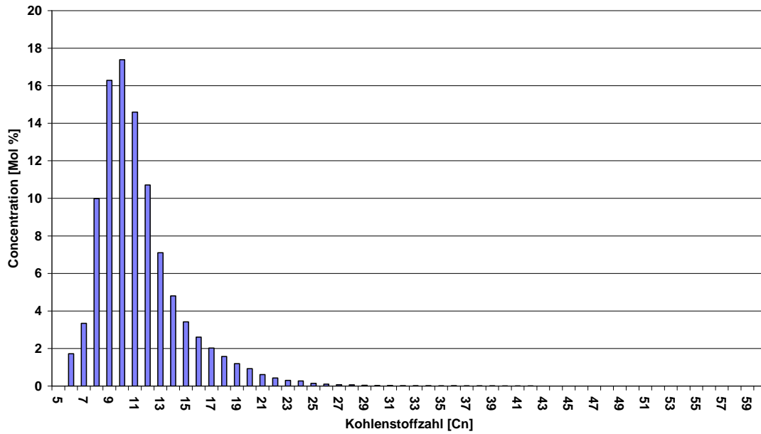
Abbildung 5.18: Produktverteilung von dem FT-Produkt im Off-gas kondensiert im Kühler; FT162 Versuch #10 (Säule 2)
