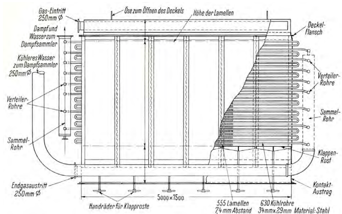
Abbildung 4.1: Industrieller Normaldruck-Festbettreaktor
