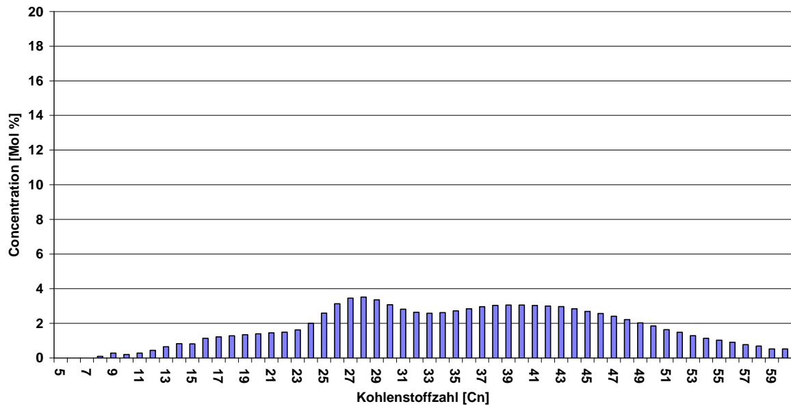
Abbildung 5.19: Produktverteilung von dem FT-Slurry im Reaktor nach dem Versuch; FT169; Versuch #10 (Säule 2)
